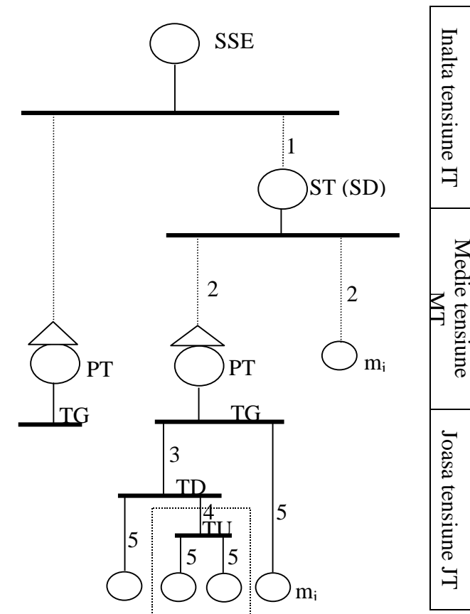
Fig. 1 - Componerea instalatiilor electrice la consumator
